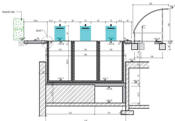
Illustration : coupe projet
