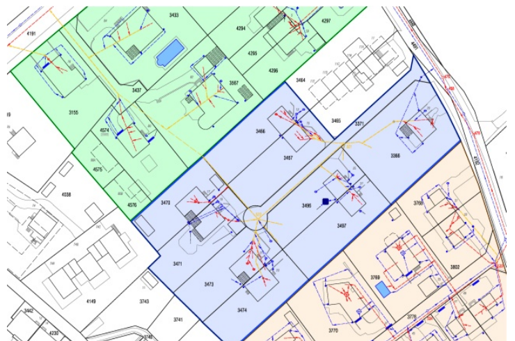
Illustration : extrait du plan global des canalisations
