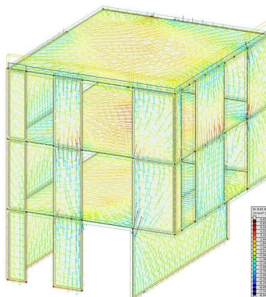
Modèle 3D Axis VM 12 - contraintes principales
